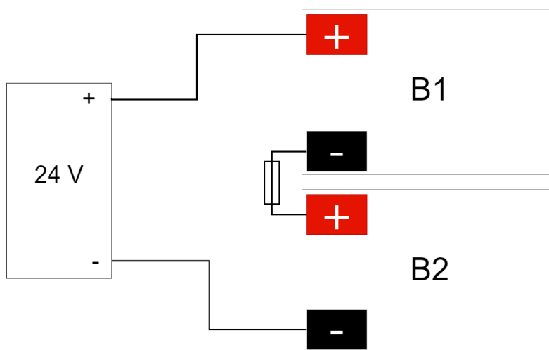
Figur 1. Kopplingschema för batterier i batteribackup
